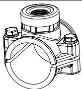
BL120-250 Injectorzadel voor 50 mm diameter buis, 1/2" draad
