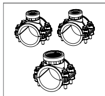
BL120-163 Vattingkit voor 63 mm diameter buis (2 zadel voor injectoren, 1 zadel voor elektrode)
