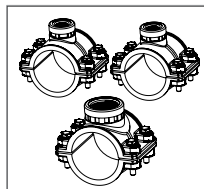
BL120-175 Vattingkit voor 75 mm diameter buis (2 zadel voor injectoren, 1 zadel voor elektrode)
